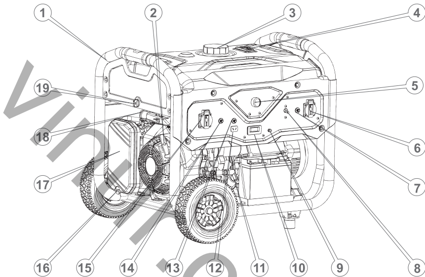
Рисунок 3. Загальний вигляд моделі «KLS 6.0 bet»
