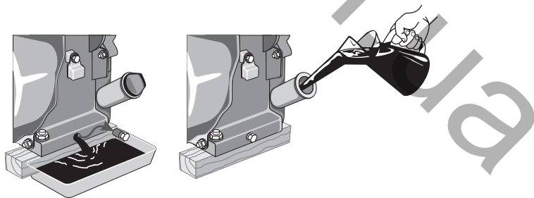
Рисунок 9. Схема заміни моторного мастила.
