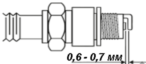
Рисунок 5. Величина зазору між електродами свічки запалювання.
