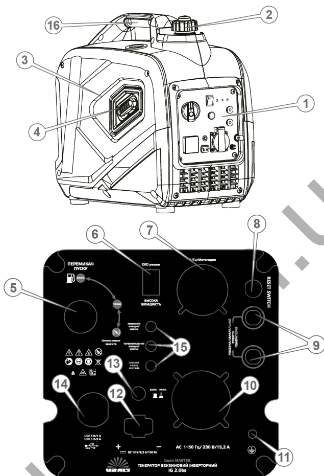
Рисунок 1. Загальний вигляд виробу та панелі керування.
