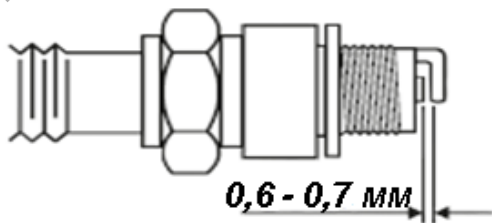
Рисунок 6. Величина зазору між електродами свічки запалювання.
