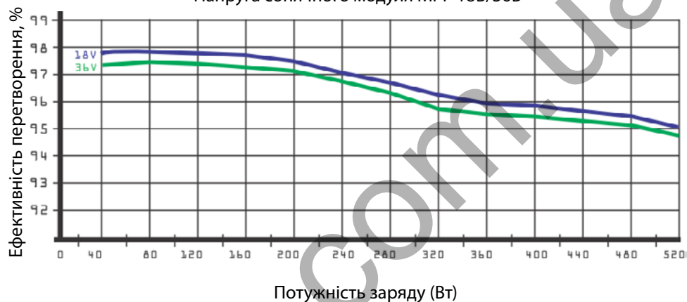
Криві ефективності перетворення 12В Напруга сонячного модуля МРР 18В/36В
