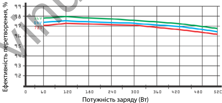
Криві ефективності перетворення 24В Напруга сонячного модуля MPP 36В/54В/72В
