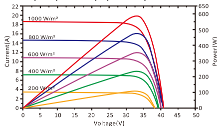
I-V характеристики при різних опромінюваннях
