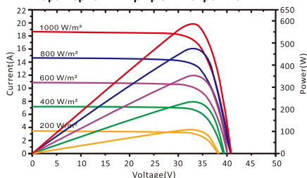
RSM120-8-590M I-V характеристики при різних опромінюваннях
