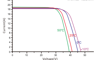
I-V характеристики при різних температурах
